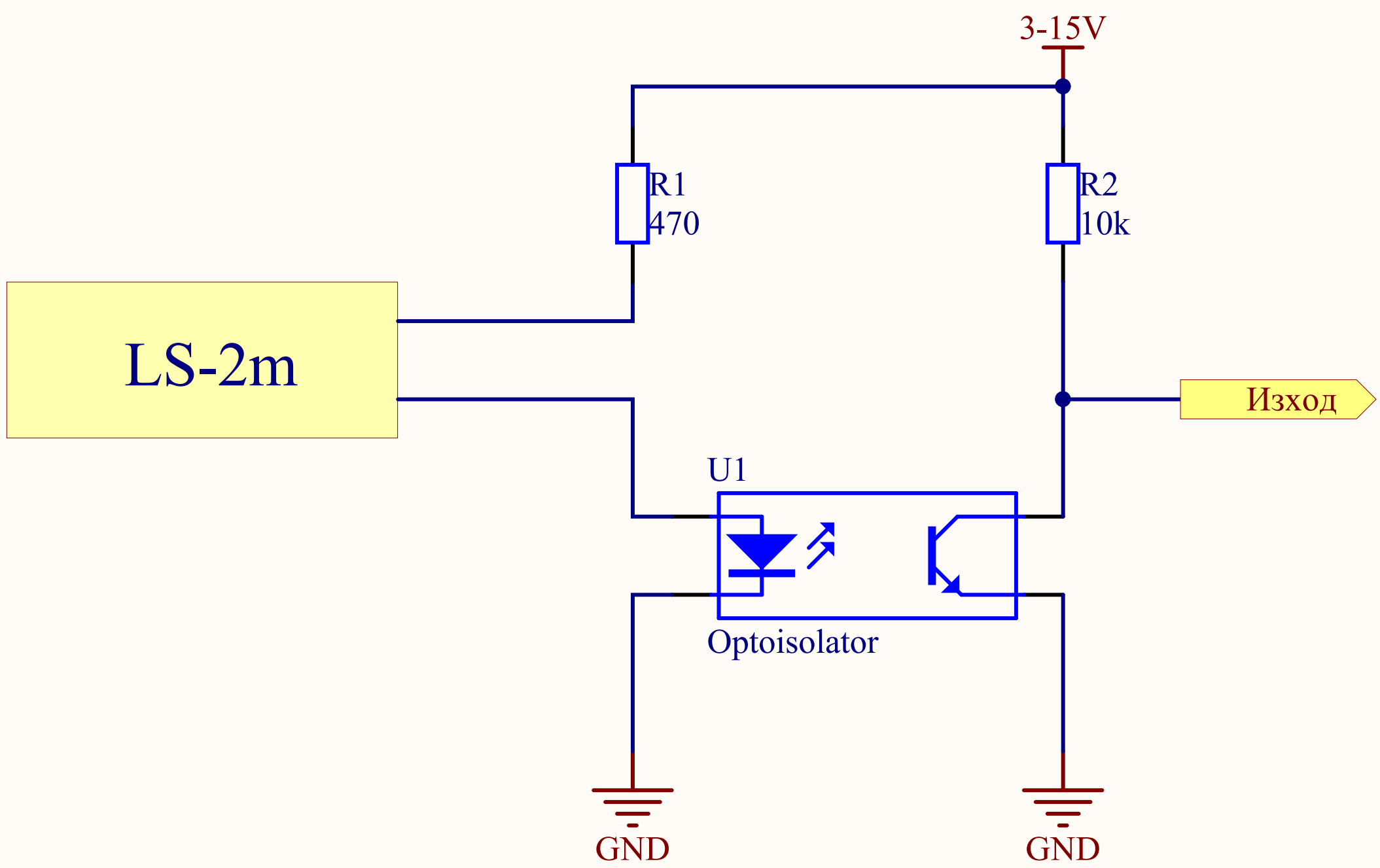
Схема на свързване с оптрон
