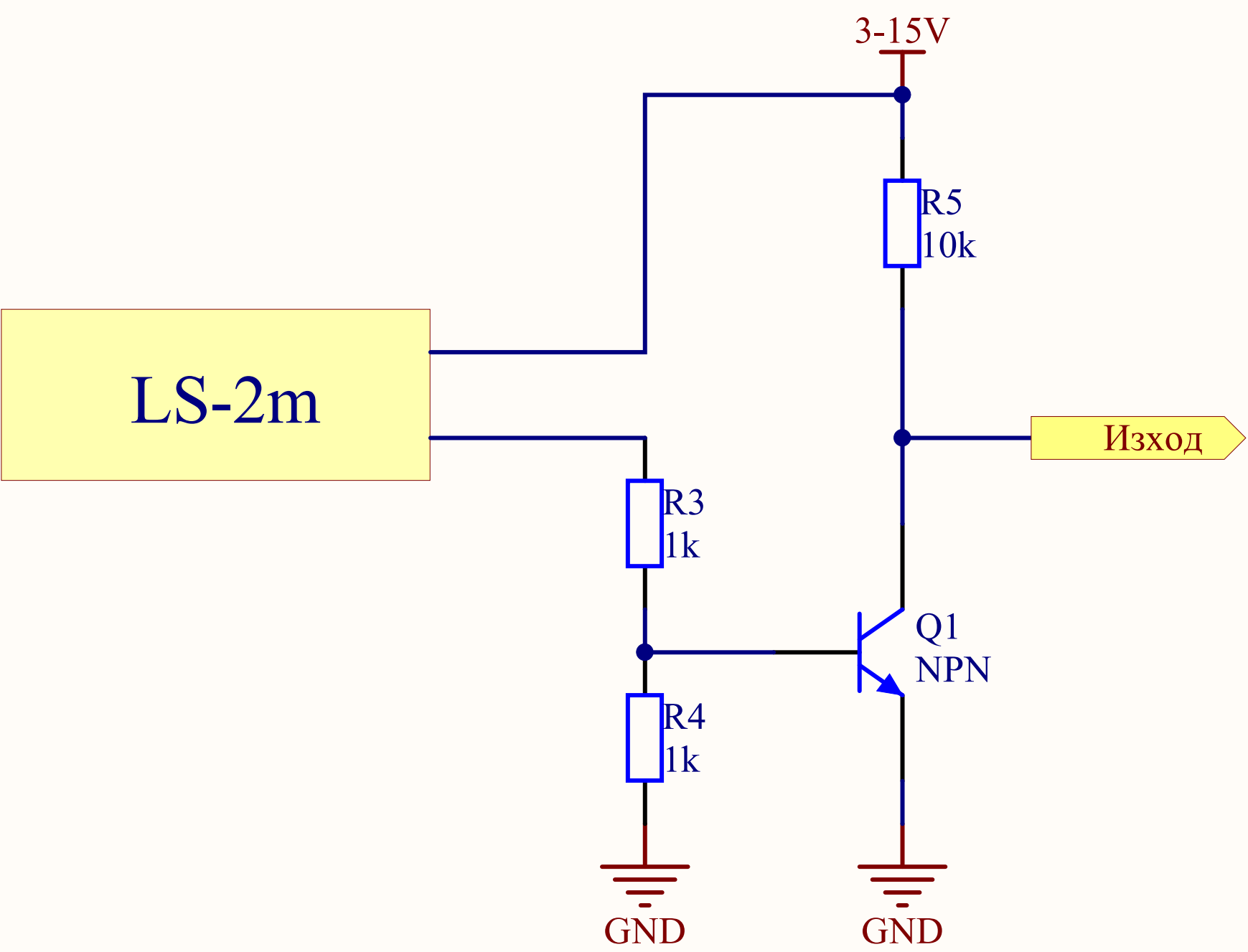
Схема на свързване с транзистор
